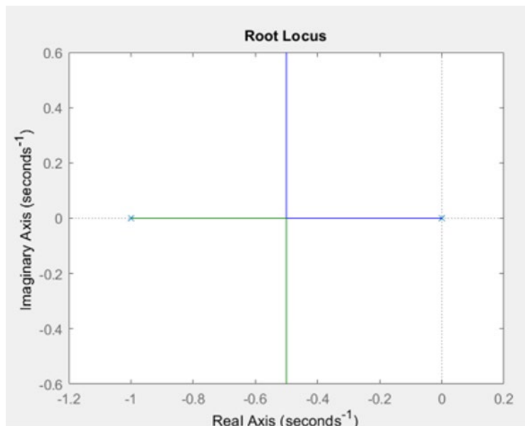
Figura 2. Lugar de las raíces de lazo abierto.
