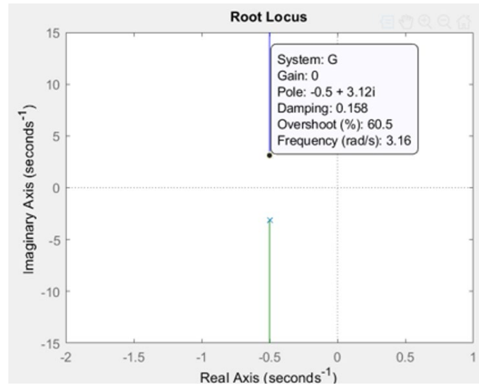
Figura 3. Lugar de las raíces de lazo cerrado.
