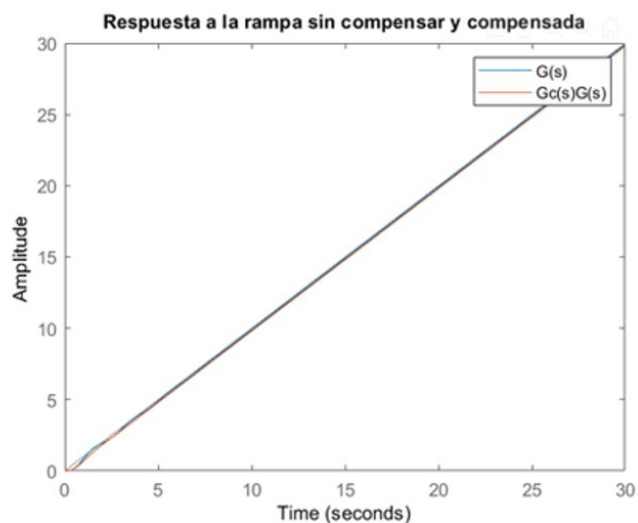
Figura 6. Gráfica de la respuesta a la rampa.
