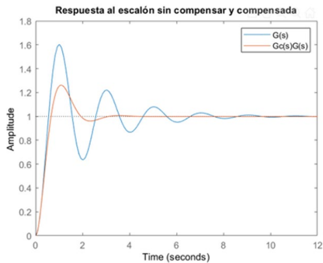
Figura 5. Gráfica de la respuesta al escalón.
