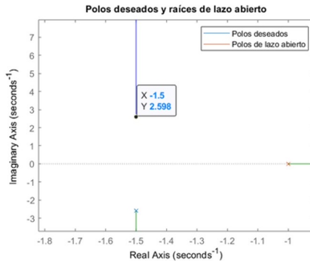
Figura 4. Lugar de las raíces de polos deseados y lazo abierto.
