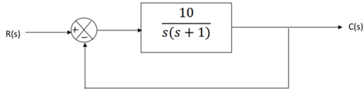
Figura 1. Sistema de control.
