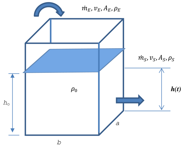
Figura 2. Tanque recuperador.
