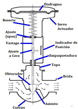
Figura 13. Elementos de una válvula de control.
