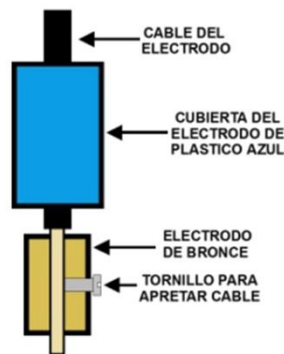
Figura 16. Electrodos.
